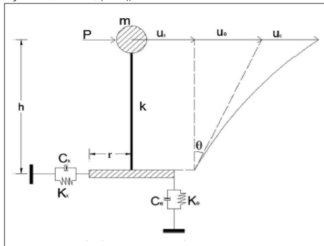
1. ábra: A síkalapozású szerkezet egyszerűsített modellje (Maravas, Mylonakis, Karabalis, (2014)).
