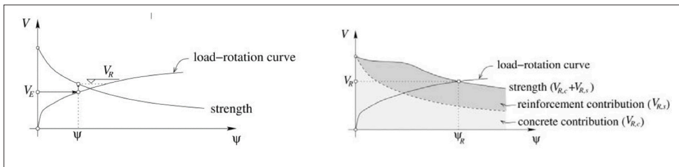
6. ábra: Erő-elfordulás (load-rotation curve) összefüggés, tönkremeneteli kritérium (strength) valamint a beton ( V_{R,c} ) és az átszűrődési vasalás részese- sedése ( V_{R,s} ) átszűrődésre vasalatlan, illetve vasalt esetben (Muttoni 2013)
