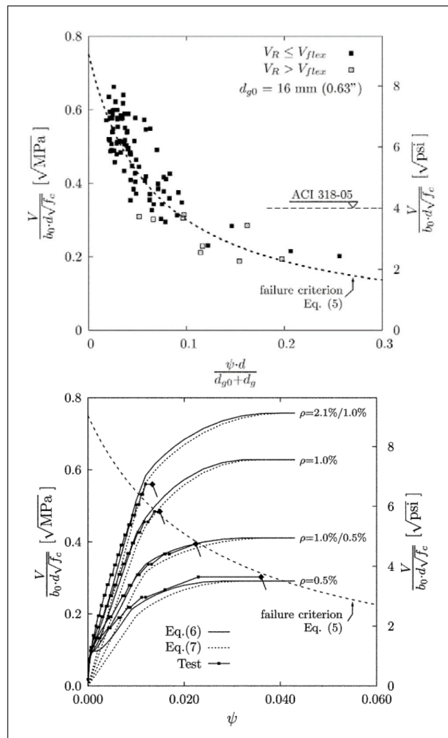
4. ábra: A hajlítási teherbírás elért (négyzet) és el nem érő (teli négyzet) próbatestek átszűrődési ellenállása a repedés tárgasságát és repedés érdességét leíró tényező függvényében (Muttoni 2008.), illetve a Kinnunen-féle kísérleti eredmények, és a számított erő-elfordulás összefüggések (pontvonal – bilineáris, folytonos-kvadrilineáris nyomtér-görbület összefüggés felhasználásával), valamint a tönkremeneteli pontokra illeszthető tönkremeneteli kritérium (Muttoni 2008.)
