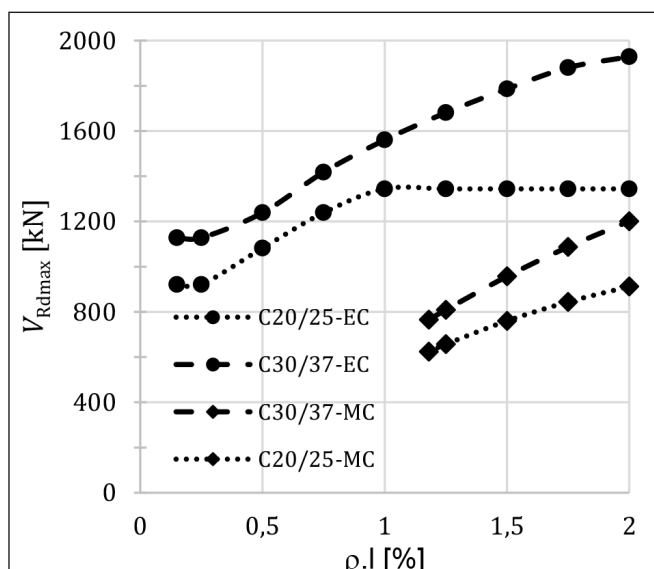
14. ábra: Felső korlátok összehasonlítása 50/50 pillér ( k_{\max}=2.5 ; k_{\text{sys}}=2.8 )
