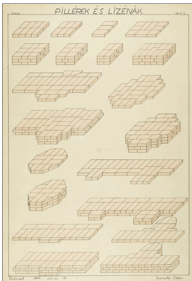
13. ábra: Susánszky Gábor rajza pillérek és lizénák téglakiosztásáról, keltezés: 1944 (forrás: Éptört. Rajzt. 103133)
