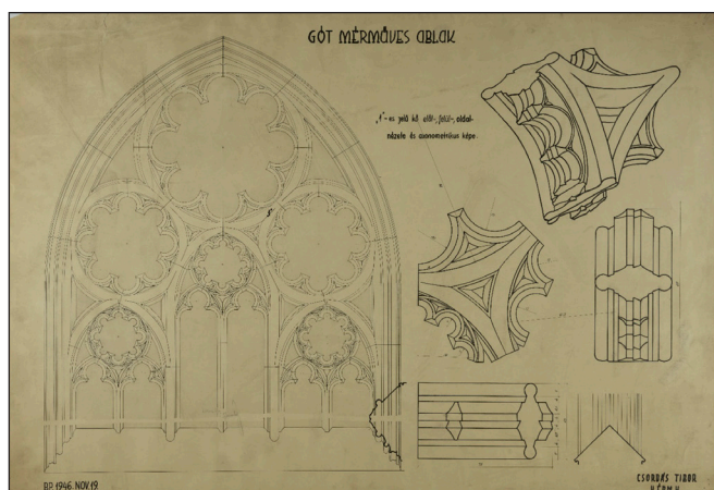
12. ábra: Csordás Tibor másodéves hallgató rajza mérműelemek szerkesztéséről, keltezés: 1946 (forrás: Éptört. Rajzt. 103322)
