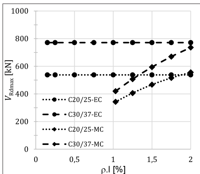
13. ábra: Felső korlátok összehasonlítása 20/20 pillér ( k_{\max}=2.5 ; k_{\text{sys}}=2.8 )
