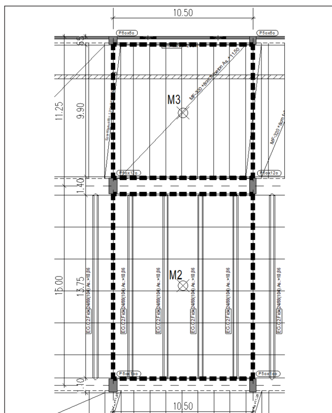
2. ábra: Probaterheléshez kiválasztott födémterület
