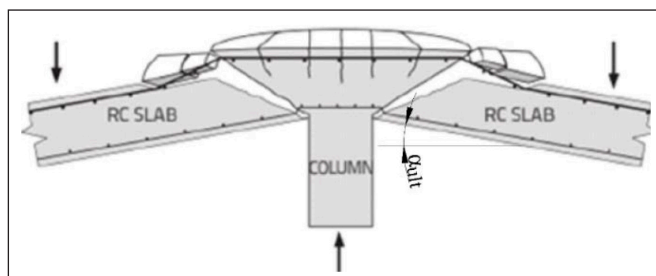
9. ábra: Az integritási vasalás működése és az \alpha_{ul} szög értelmezése (Bartolac, Damjanovic és Ivan 2015.) ábrája nyomán
