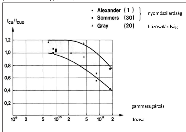
8. ábra: A gammasugárzásnak kitett beton nyomó-, és húzószilárdsága ( f_{cu} ) a nem kitett kontroll próbatestek szilárdságának ( f_{cu0} ) arányában (Hilsdorf-Koch-Kropp, 1978)
