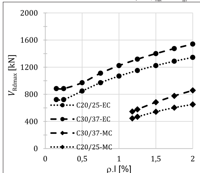
12. ábra: Felső korlátok összehasonlítása 50/50 pillér ( k_{\max}=2.0 ; k_{\text{sys}}=2.0 )
