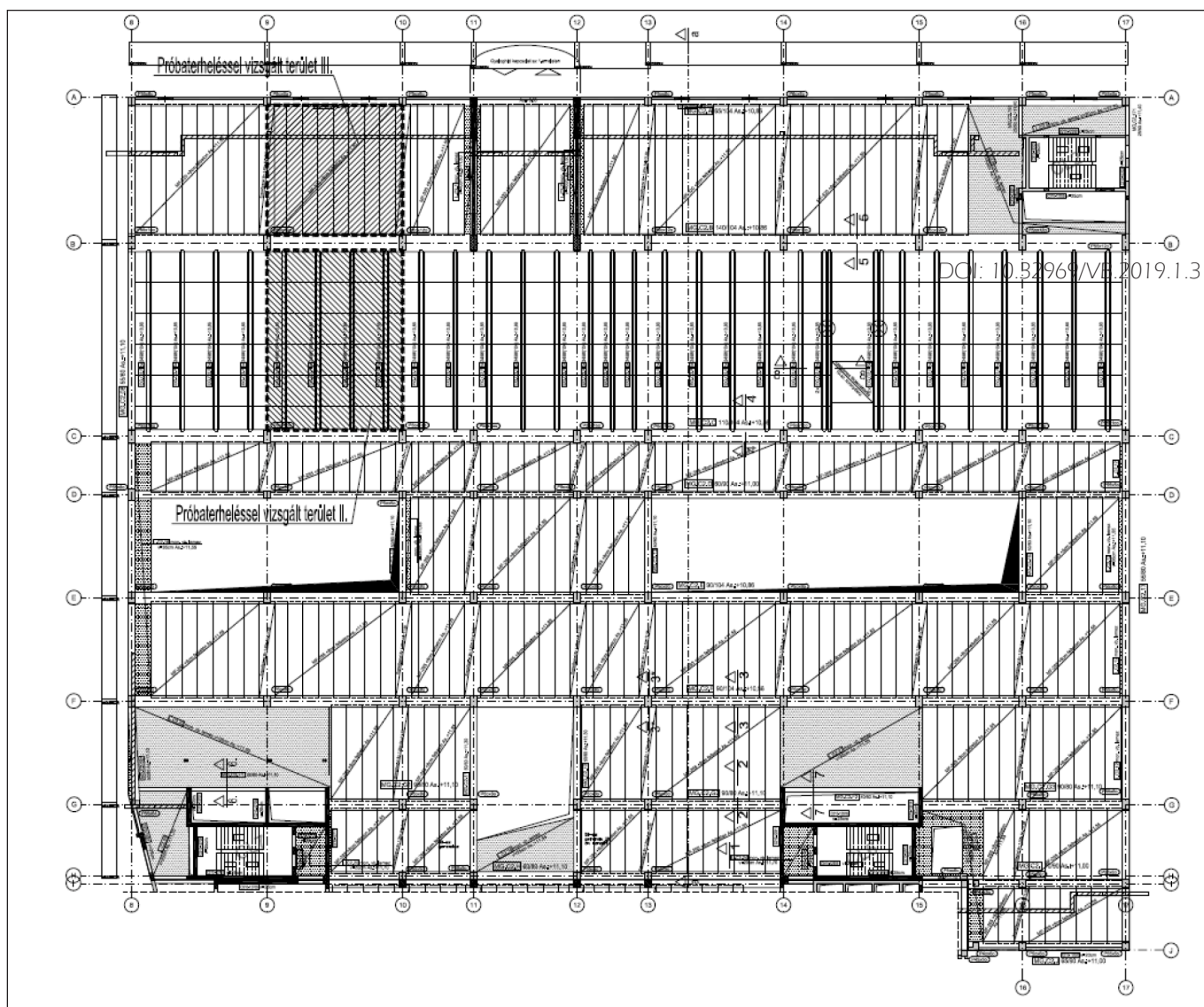
1. ábra: Előre gyártott elemekkel kialakított födémrendszer
