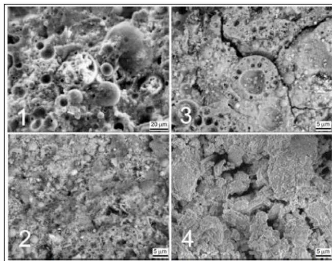
3. ábra: Pernye és portlandcement keverékből készült cementpép mikrostruktúrájának változása gamma sugárzás hatására 1. 0 MGy; 2. 290 MGy; 3. 466 MGy; 4. 1188 MGy. (Lowinska-Kluge, Piszora, 2008) (A gray (jele: Gy, ejtése: gréj) az elnyelt sugárdózis , a fajlagos (közölt) energia SI származtatott egysége . MGy=megagréj)
