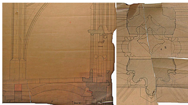
9. ábra: Szerkezeti részletek a prágai székesegyház támvívet és kötegpillérét ábrázoló rajzokról, keltezés: 1905 (forrás: Éptört. Rajzt. 105987, 105985)
