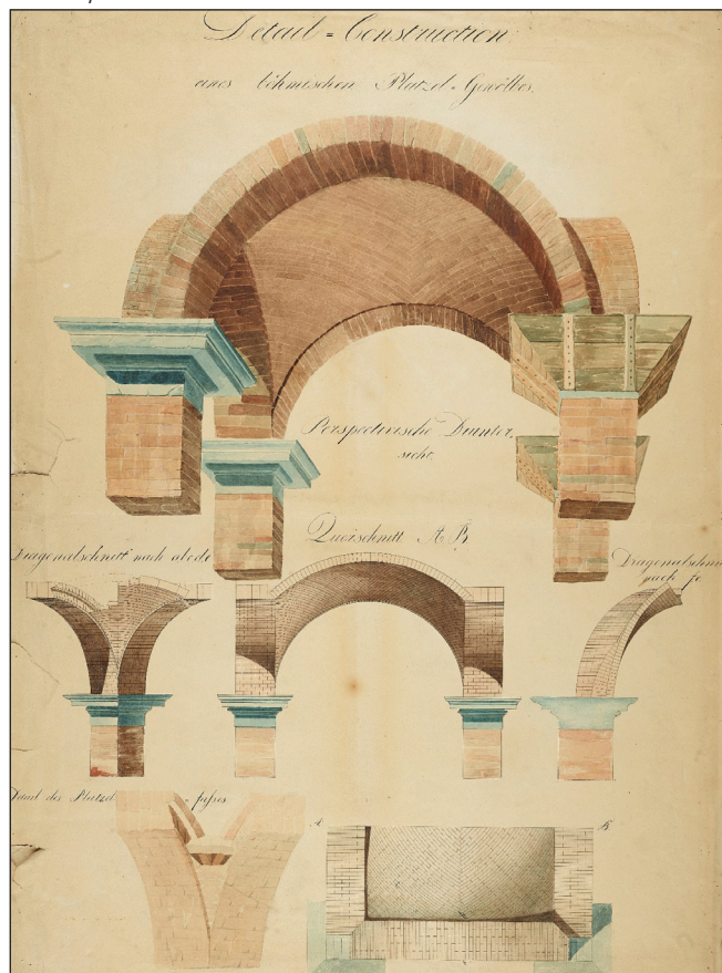
3. ábra: Csehsüveg boltozat részletes szerkezeti rajzai perspektívában, metszetekkel és alaprajzban ábrázolva. Felirat: „Detail-Construction eines böhmischen Platzel-Gewölbes”, keltezés: s.a. (forrás: Éptört. Rajzt. 105862)
