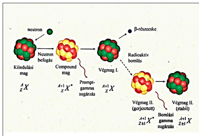
2. ábra: A neutron hatása adott molekulán (Szentmiklósi-Katovszky, 2012) Az elnyelt sugárzás gyengíti a betonszövetet
