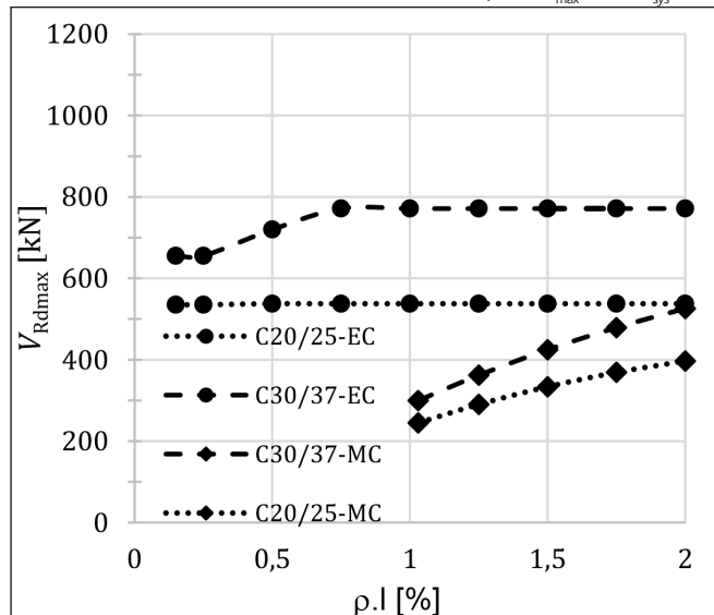
11. ábra: Felső korlátok összehasonlítása 20/20 pillér ( k_{\max}=2.0 ; k_{\text{sys}}=2.0 )
