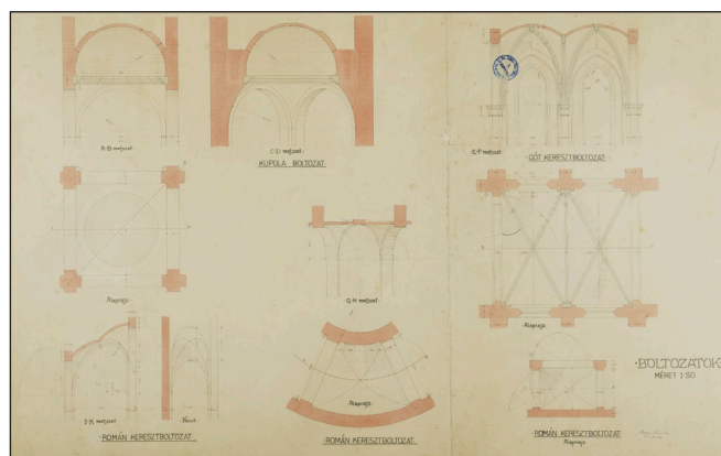
11. ábra: Möller Károly hallgatói rajza középkori boltozatok szerkezeti kialakításáról, keltezés: s. a. [1916 körül] [forrás: Éptört. Rajzt. 102328]
