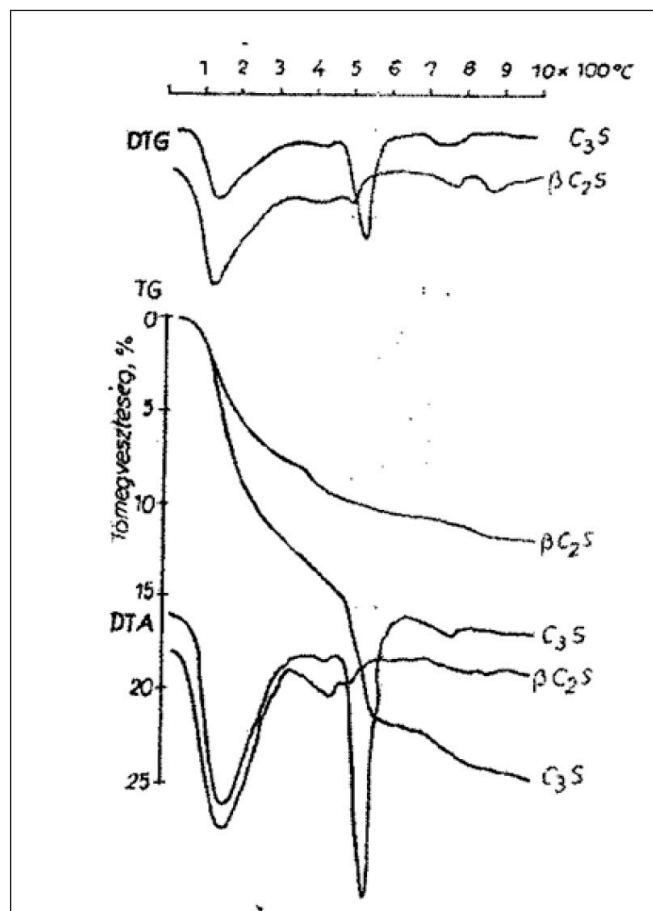
6. ábra: A megszilárdult portlandcement két legfontosabb szilárdsághordozójának derivatogramja (C3S és βC2S). A TG görbén észlelhető, hogy 200 °C-ig jelentős a tömegvesztés (Balázs, 2001)
