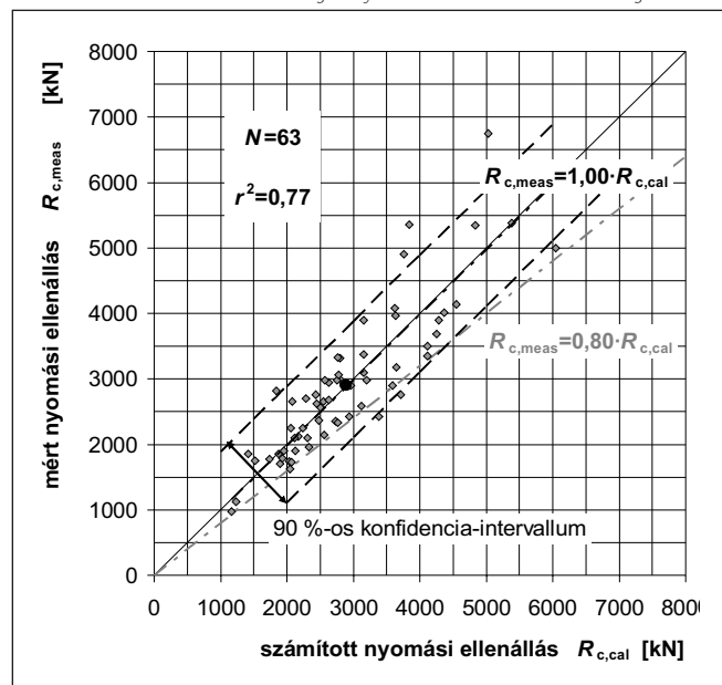
5. ábra: A mért és számított teljes nyomási ellenállások korrelációja
