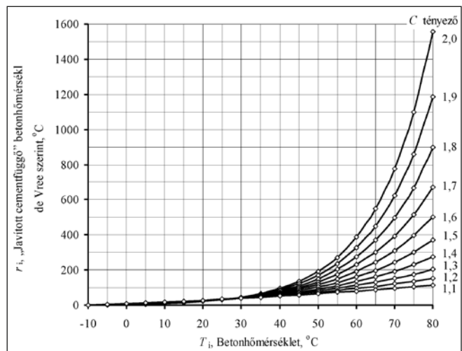
15. ábra: „Javított cementfüggő” (korrigált) betonhőmérséklet de Vree szerint ( r_i ) a betonhőmérséklet ( T_i ) és a cement hőérzékenységét kifejező C tényező függvényében, a (8) összefüggés alapján
