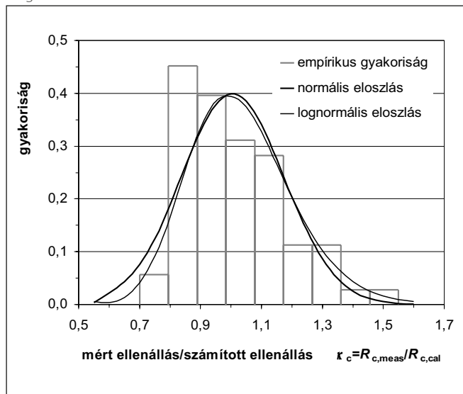
4. ábra: A mért és számított nyomási ellenállások viszonzszámának gyakorisága
