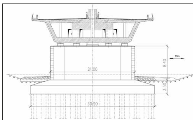
1. ábra: A mederpillér az indítózömmel
