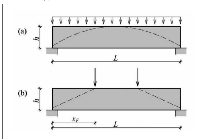
4. ábra: Vizsgált teheresetek. Egyenletesen megosztó teher (a) és a két koncentrált erő (b).
