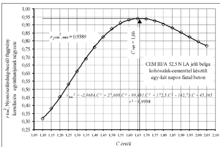
20. ábra: A belga CRIC-OCCN kísérleti eredmények értékelése a holland CEMU-féle módszerrel. A példa szerinti C_{opt} érték meghatározása ötödfokú polinommal. Vermeersch (2005) diplomamunkája után
