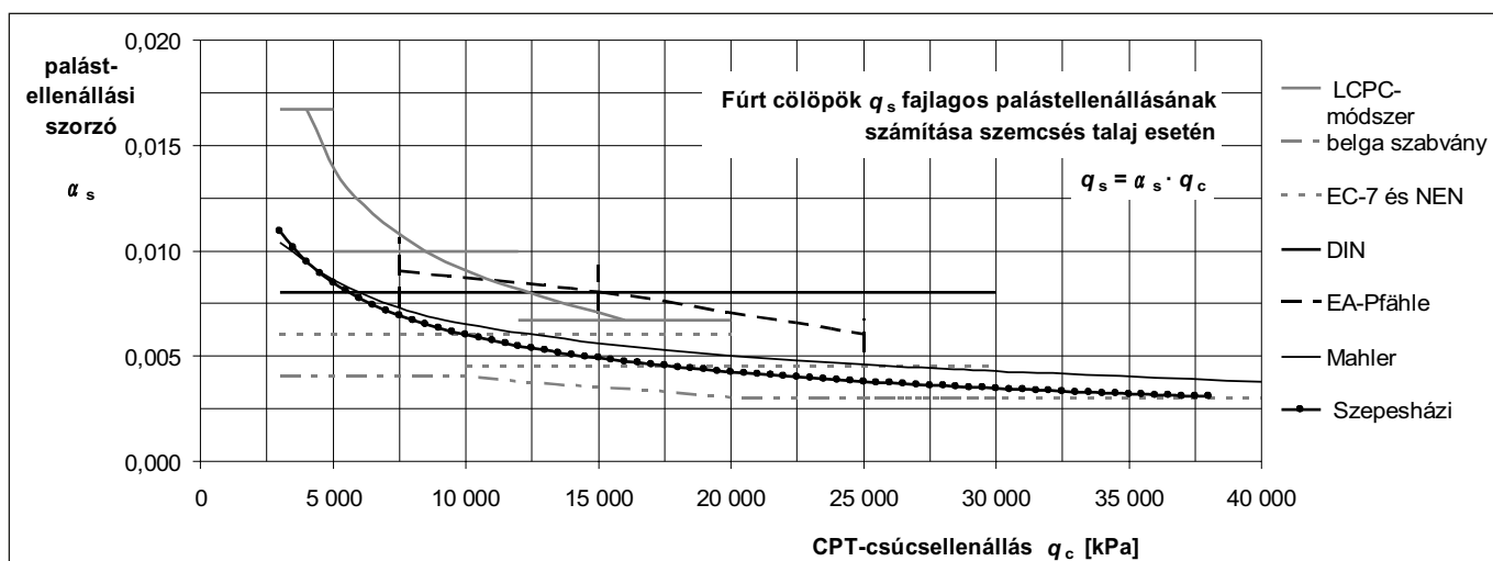
2. ábra: A szemcsés talajok esetén alkalmazható palástellenállási szorzók összevetése
