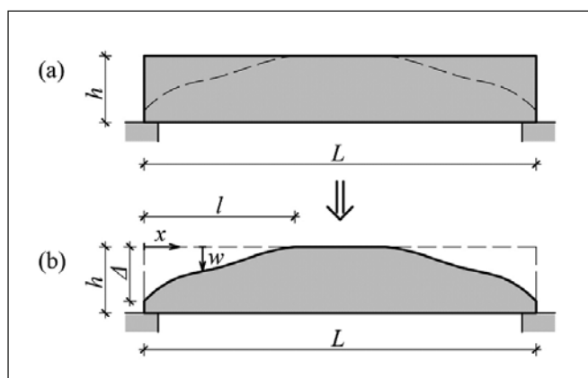
3. ábra: A gerenda fiktív levágása. Az eredeti gerenda (a) és a számításkor figyelembe vett modell (b).
