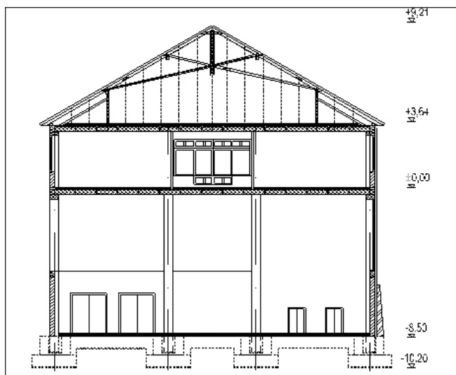
3. ábra: Keresztmetszet
