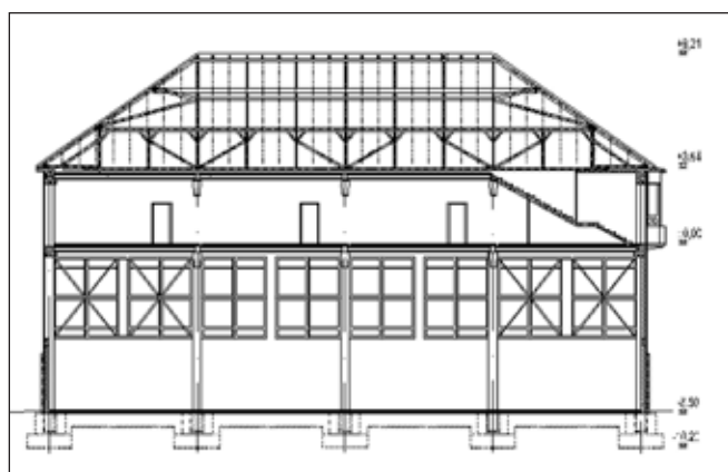
4.ábra: Hosszmetszet
