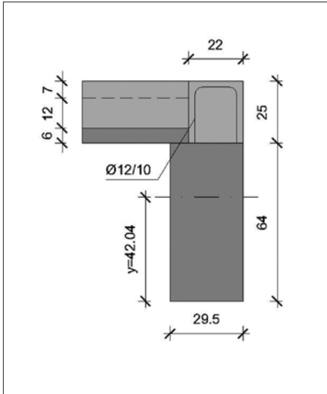
13. ábra: Födémgerenda
