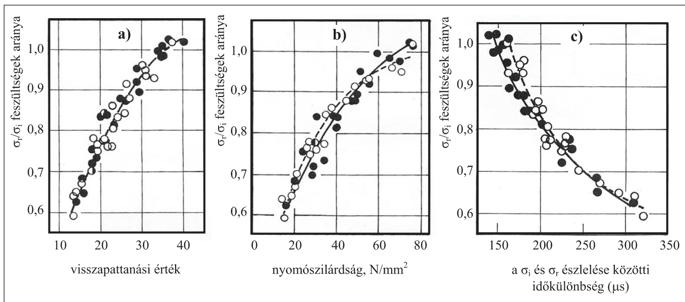
3. ábra: Összefüggések a visszapattanási érték, a nyomószilárdság és a mechanikai hullámok egyes paramétereinek között (Akashi, Amasaki, 1984)
