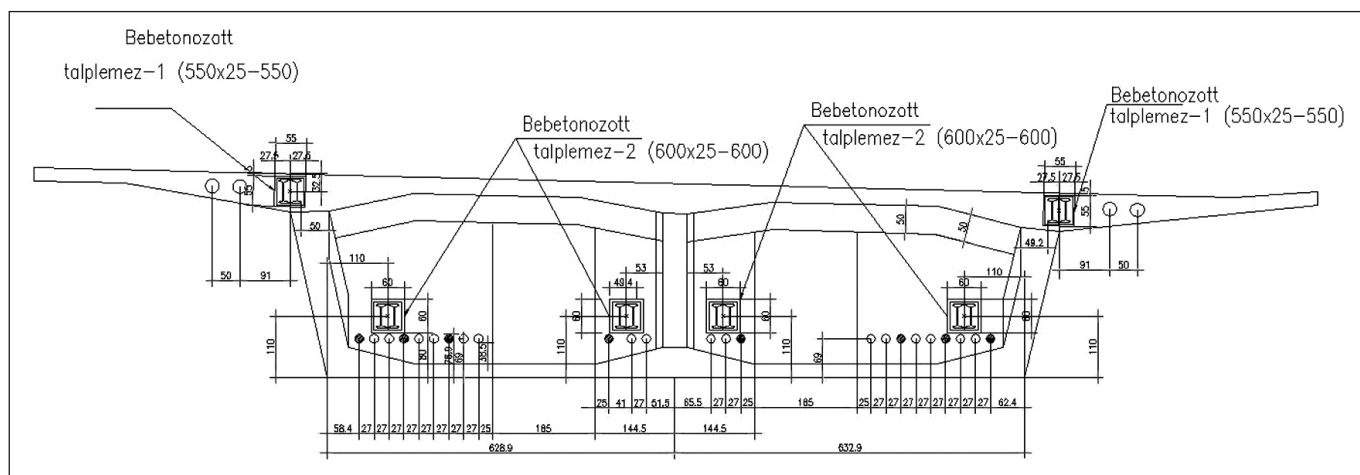
12. ábra: A kitámasztó dúcok kiosztása a híd keresztmetszetében
