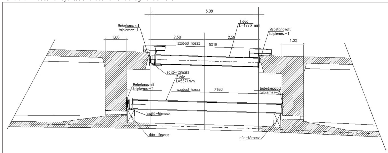
13. ábra: A dúcok elhelyezése az utolsó zömök diafragma-falai között
