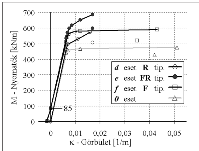
6. ábra: A teherbírás határállapothoz tartozó pontok (az anyagjellemzők tervezési értékével számítva), és nyomaték-görbület diagramok (az anyagjellemzők karakterisztikus értékével számítva), a 3. táblázatban leírt, azonos megerősítés-merevséget, és feszítőerőt alkalmazó megerősítésekkel
