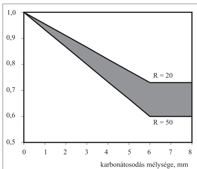
7. ábra: Korrekció a karbonátosodás mélységének figyelembe vételére a JGJ/T23-2001 jelzetű kínai nemzeti szabvány javaslata szerint, R = 20 – 50 visszapattnási értékek között (Proceq, 2003)
