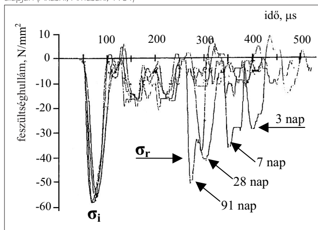
4. ábra: Mechanikai hullámok időbeli alakulása, egy v/c=0,70 víz-cement tényezőjű betonon 3, 7, 28 és 91 napos korban mért vizsgálati eredmények alapján (Akashi, Amasaki, 1984)
