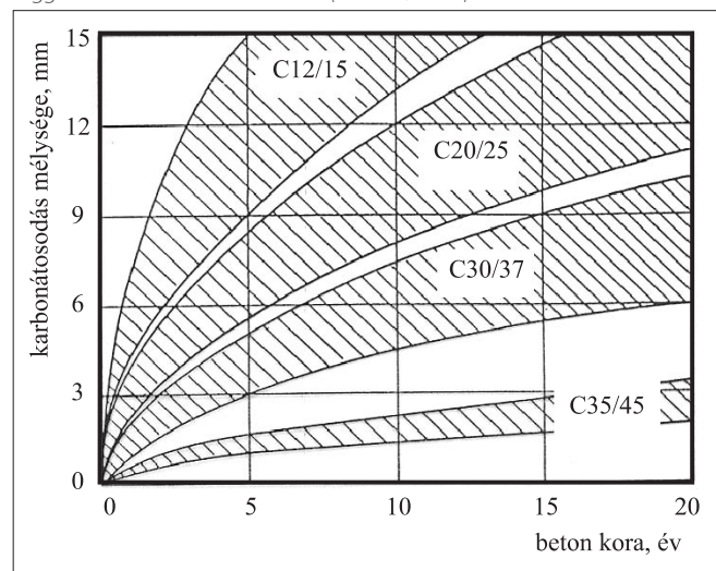
6. ábra: A karbonátosodási mélység és a beton nyomószilárdság összefüggésének sematikus ábrázolása (Bindseil, 2005)
