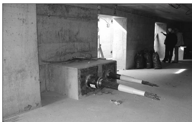
7. ábra: Erőmérő henger a kábelek lehorgonyzásánál
