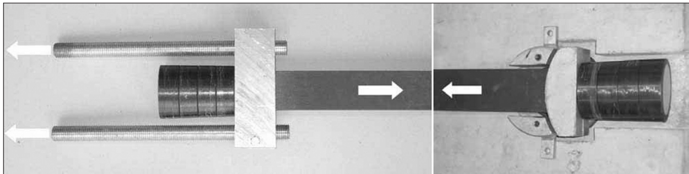
3. ábra: StressHead lehorgonyzási lehetőségek: állítható – fix (StressHead, 2005)
