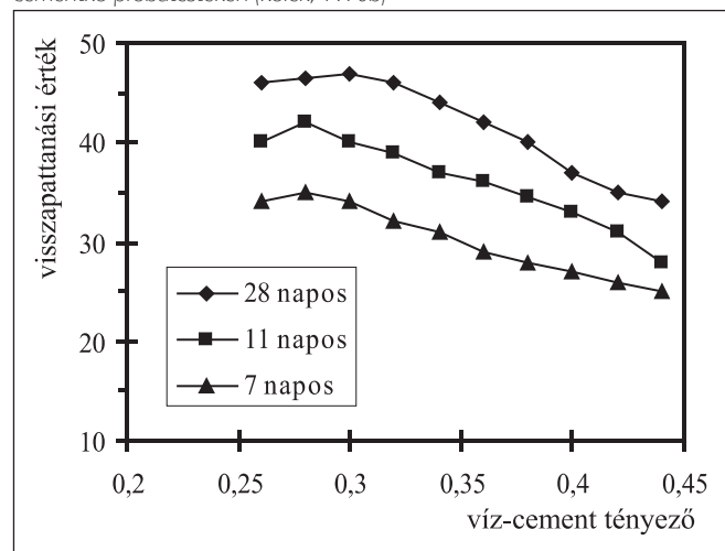
1. ábra: Schmidt-kalapácsos visszapattnási értékek megszilárdult cementkő próbatesteken (Kolek, 1970b)
