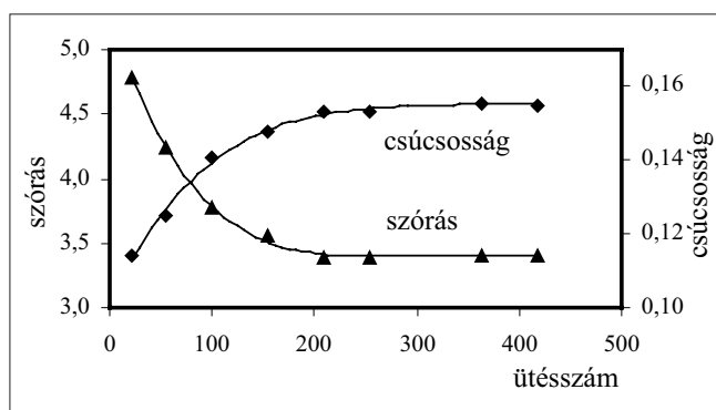
8. ábra: Matematikai statisztikai jellemzők (szórás és csúcsosság) aszimptotikus viselkedése egy vasbeton fal Schmidt-kalapácsos vizsgálati eredményei alapján
