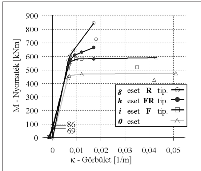
7. ábra: A teherbírás határállapothoz tartozó pontok (az anyagjellemzők tervezési értékével számítva), és nyomaték-görbület diagramok (az anyagjellemzők karakterisztikus értékével számítva), a 4. táblázatban leírt, azonos merevségnövelő-hatást elérő megerősítésekkel
