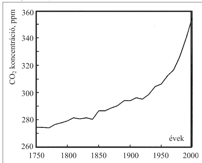
12. ábra: A légkör CO 2 koncentrációjának növekedése az elmúlt 250 évben (Yoon et al, 2007)
