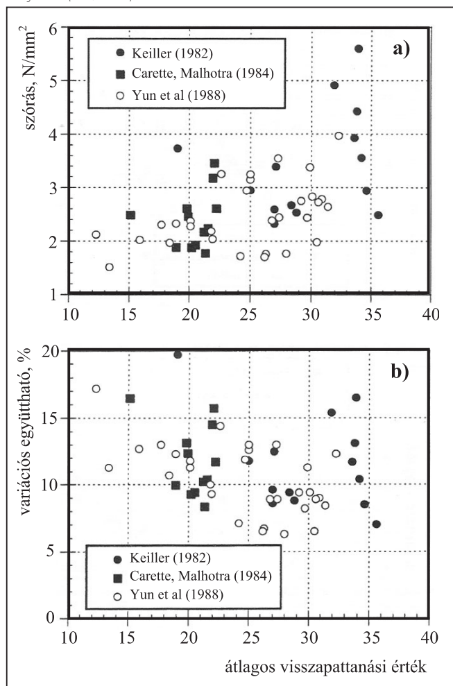
10. ábra: Schmidt-kalapácsos visszapattnási értékek a) vizsgálaton belüli szórása, és b) variációs együtthatója, az átlagos visszapattnási érték függvényében (ACI, 2003).
