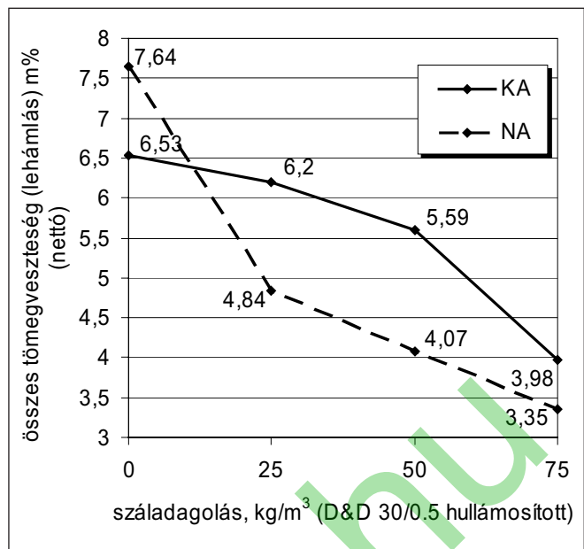
3.a ábra: Tömegveszteségek 32 ciklusú forgatásos fagyasztás után a szártartalom függvényében. (A-módszer, a fagyasztási ciklusok után további 3 hónapig lehámlott tömegekkel együtt) (Erdélyi, Borosnyói, 2005b)
