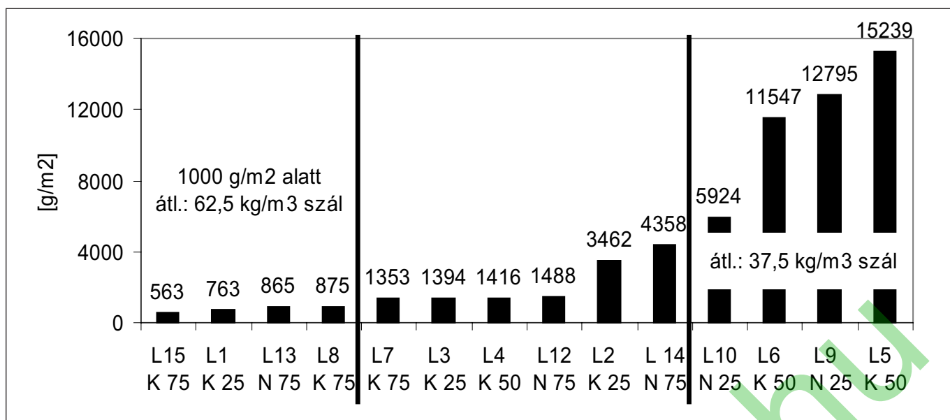
11. ábra: Összes normalizált lehámlás növekvő sorrendben 56 ciklusra
