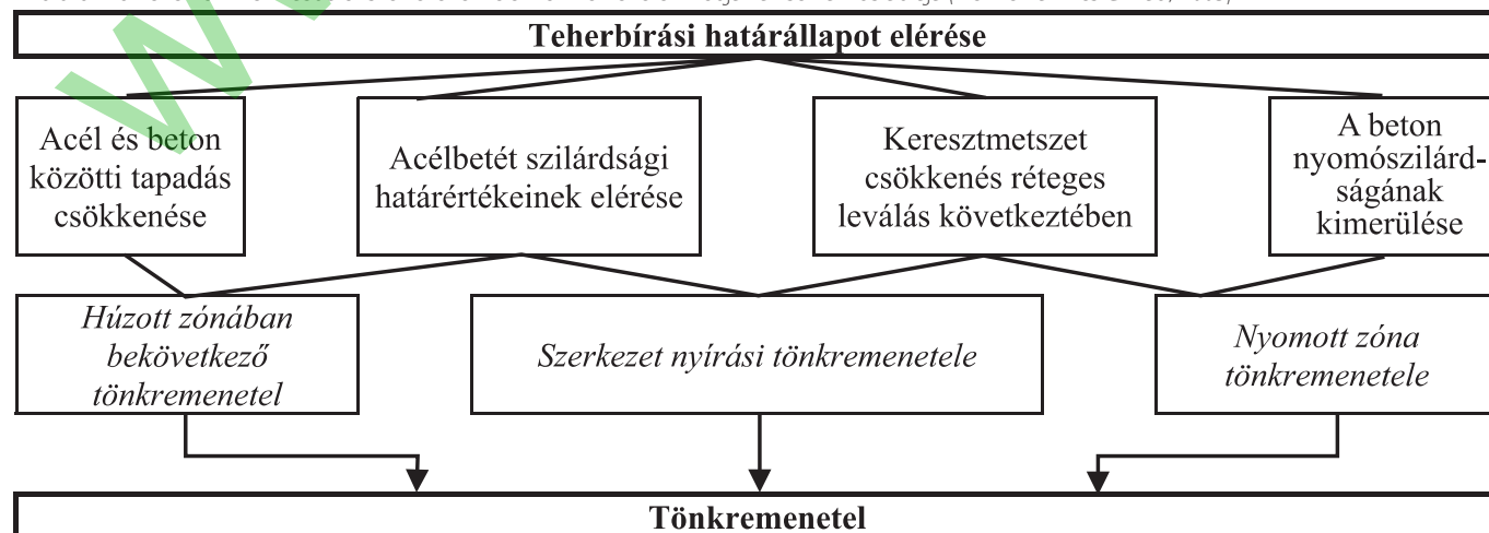
2. ábra: Tűzterhekre kitétt vasbetonszerkezet elméleti tönkremeneteli módjainak sematikus ábrája (Blennemann és Girmau, 2005)
