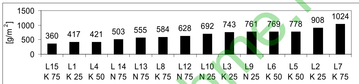
10. ábra: Összes normalizált lehámlás növekvő sorrendben 28 ciklusra
