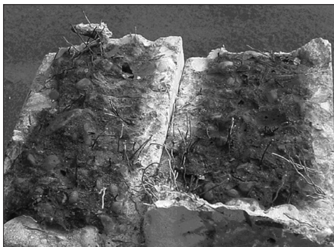
12. fénykép. 28 napig vízben, utána 10 évig laborlevegőn tárolt vízzáró-sági próbatest, elhasítva: a szálak matt fémfényűek (megjegyzés: a középső, sötétebb tónusú tartományok fenolftalein pozitívak)
