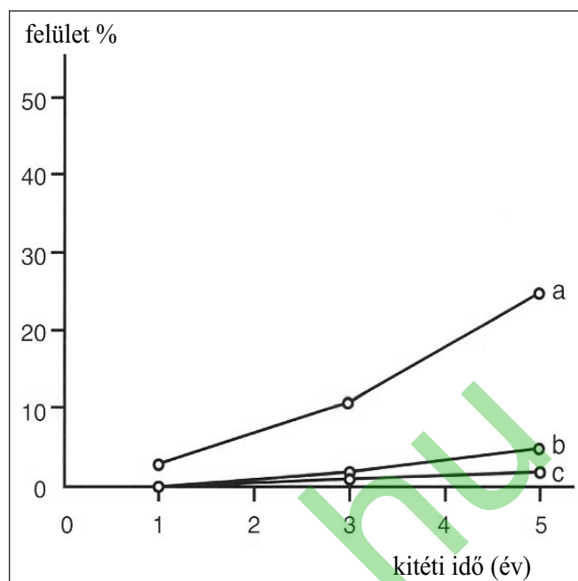
7. ábra: 10 mm átmérőjű betonacél felületi korróziója háromféle betonban (Bekaert, 1988)
