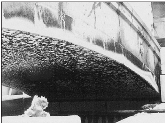
17. ábra: Kísérleti elrendezés és égetett betontübbing (Blennemann és Girnau, 2005)
