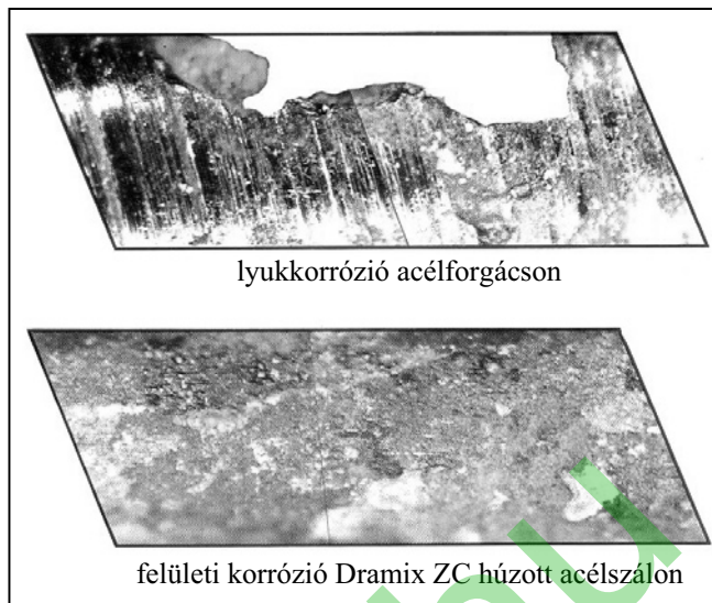
6. ábra: Forgácsolt, illetve húzott acélszál korróziója betonban (0,4-0,5 mm repedésszélességig előreperesztett acélszálak beton próbatestek vizsgálata, az Nr. X41-es nemzetközi formula szerinti sós környezetben) (Bekaert, 1988)
