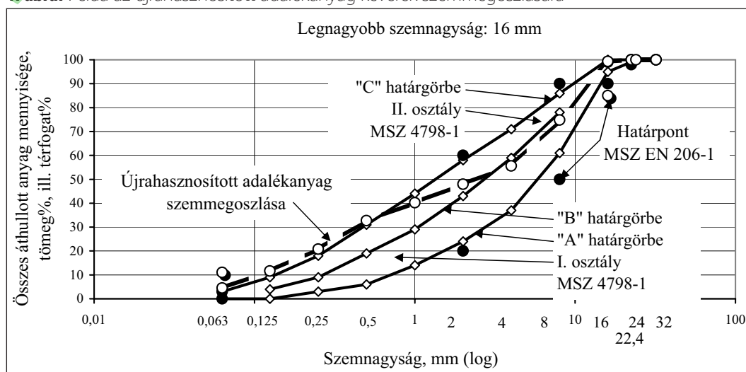
4. ábra: Példa az újrahasznosított adalékanyag keverék szemmegoszlására
