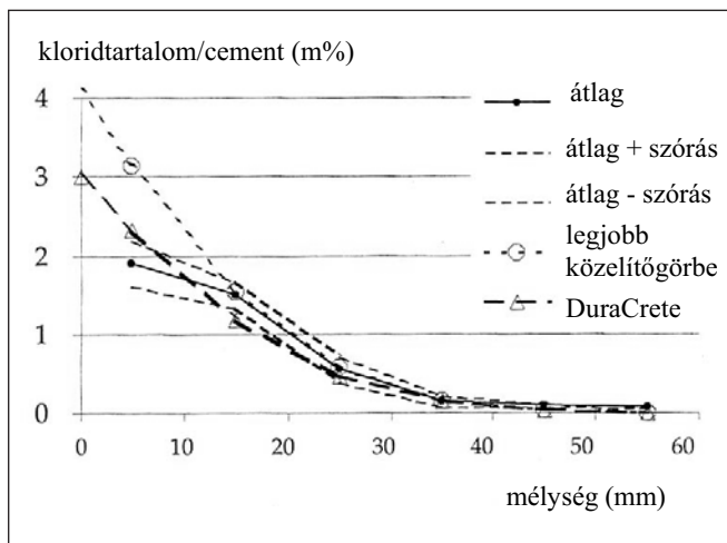
2. ábra: A klorid-behatolás mértéke (holland tengeri zsílip betonja) (Polder, Rooij, 2005)
