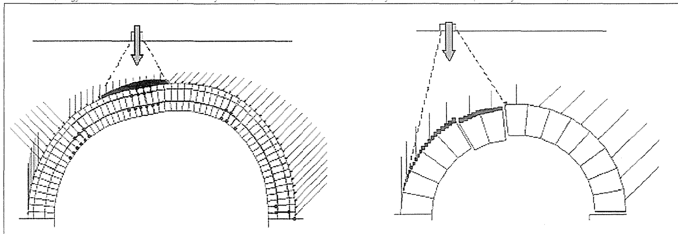
5. ábra: Boltozatok mértékadó tönkremeneteli mechanizmusai a 'merev-blokk' módszer szerint a) négycsuklós mechanizmus (5,70m nyílású híd) b) nyírási tönkremenetel (2,00m nyílású áteresz)
