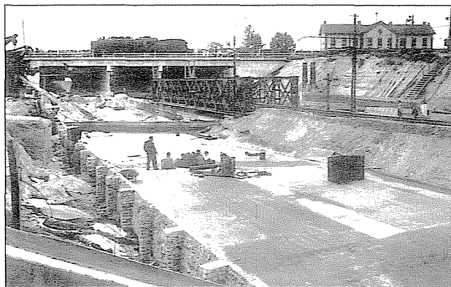
23. ábra: A Béke úti aluljáró építési munkálatai
