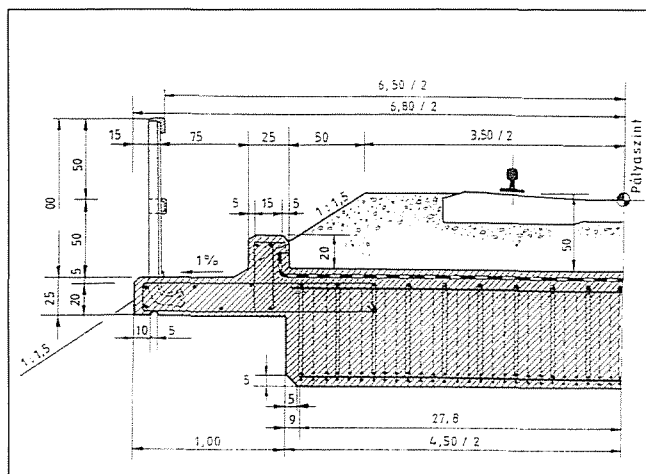
14. ábra: Ágyazátvezetéses vasbeton lemezhíd keresztmetszeti elrendezése
