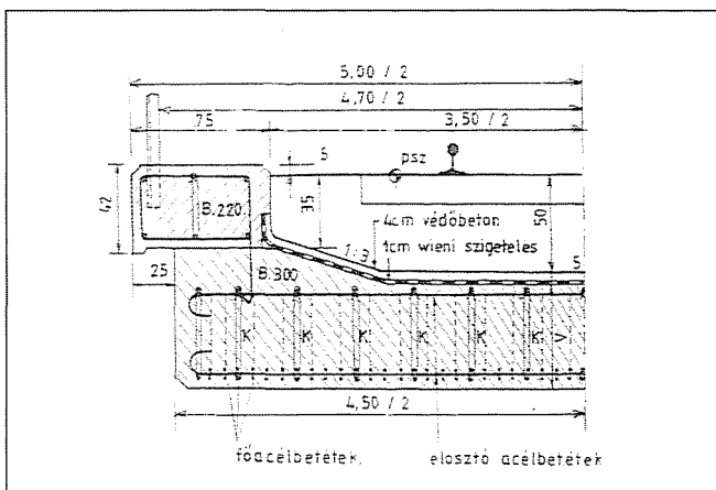
12. ábra: Az 1953. évi mintaterv szerinti vasbeton teknőhid áthidalószerkezete
