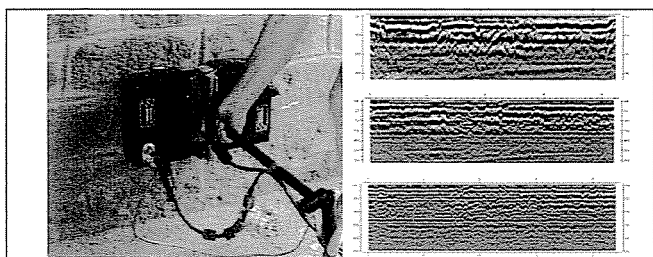
9. ábra: Vizsgálat georadarral - radarképek (felmenő fal vizsgálata különböző frekvenciájú antennákkal)
