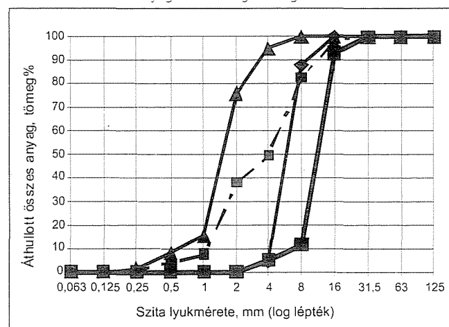
13. ábra: Az adalékanyagok szemmegoszlási görbéi
