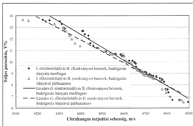
4. ábra: A I. (öntömörödő) és II. (szokványos) jelű betonkeverékek betonjainál a lineáris összefüggés (rendezett eredményeken) a terjedési sebesség és a teljes porozitás között a bedolgozás irányára merőleges és a bedolgozás irányával párhuzamos ultrahangos vizsgálat esetén
