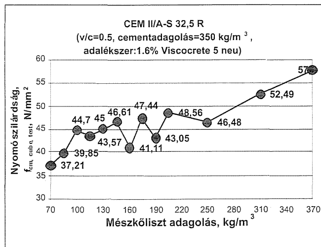
4. ábra: A mészkőliszt adagolás hatása a nyomószilárdságra
