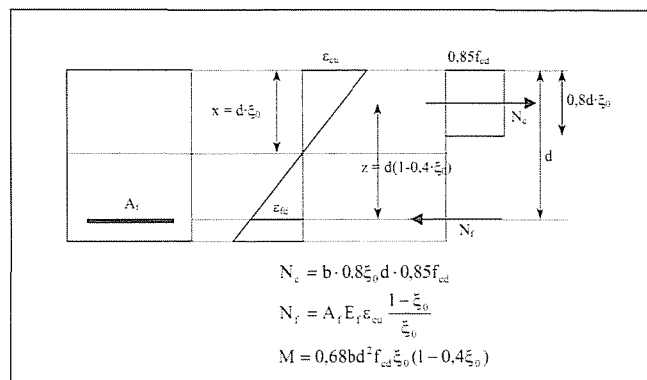
6. ábra: Inhomogén keresztmetszet belső erői
