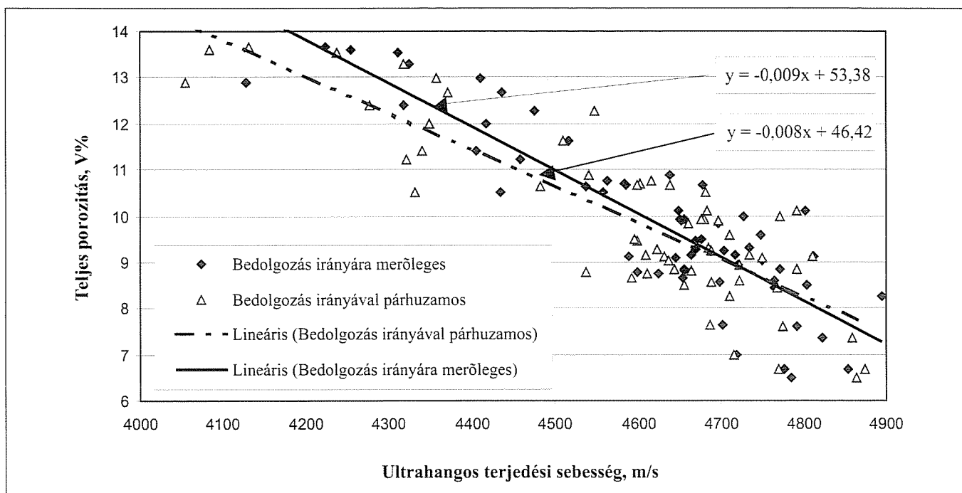
3. ábra: Lineáris összefüggés a terjedési sebesség és a teljes porozitás között a bedolgozás irányával párhuzamos és a bedolgozás irányára merőleges ultrahangos vizsgálat esetén
