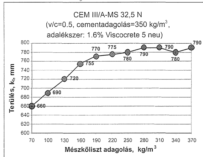
9. ábra: A mészkelet adagolás hatása a konzisztenciára
