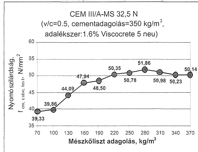
10. ábra: A mészkelet adagolás hatása a nyomószilárdságra
