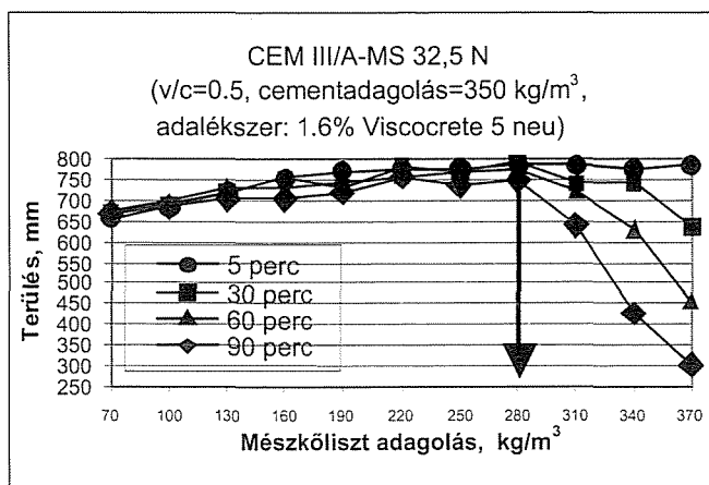
11. ábra: A konzisztencia eltarthatóság a mézkelet adagolás függvényében
