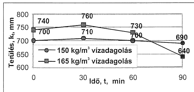
1. ábra: Az öntömörödő beton eltarthatóságának vizsgálata konzisztenciameéréssel
