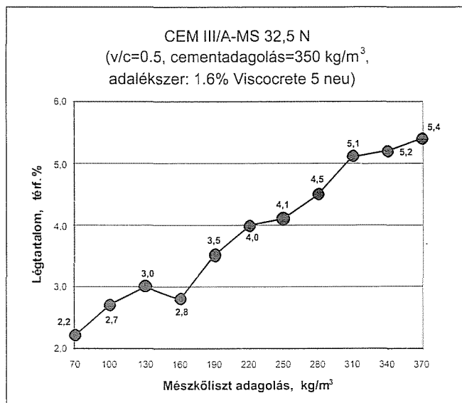
12. ábra: A mézkelet adagolás hatása a légtartalomra
