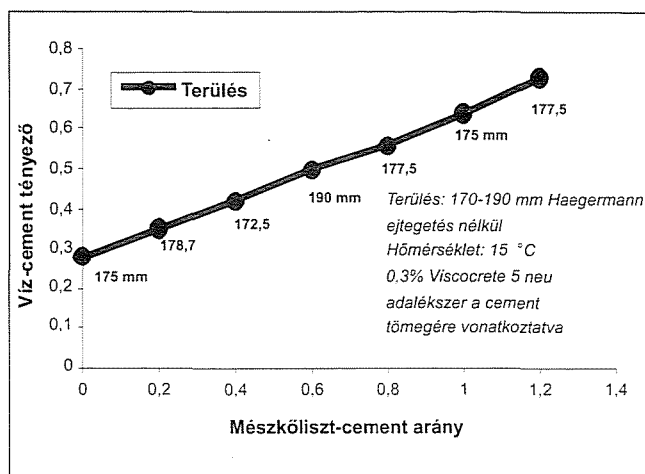
16. ábra: A mészkőliszt vízigényének alakulása azonos konzisztencia esetén
