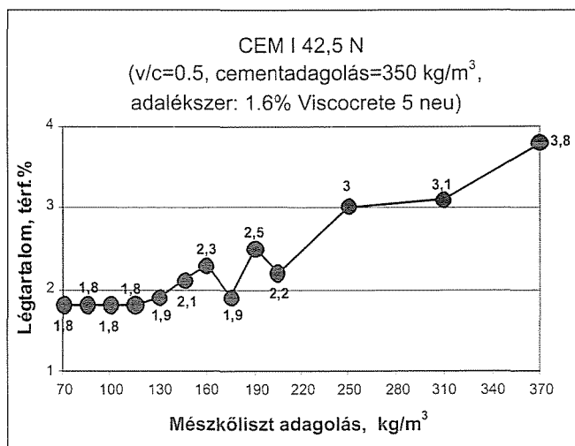
8. ábra: A friss beton légtartalmának változása a mészkelet tartalom függvényében
