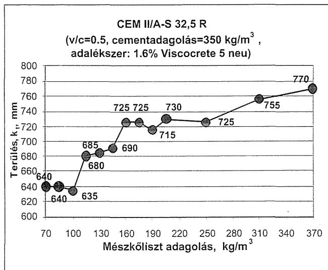
3. ábra: A mészkőliszt adagolás hatása a konzisztenciára
