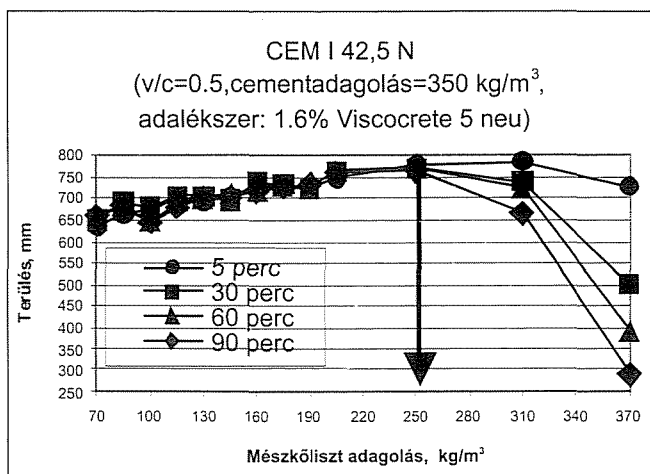
7. ábra: A friss beton konzisztenciájának és eltarthatóságának változása a mészkelet adagolás függvényében
