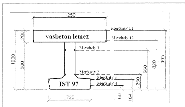
2. ábra: Az IST 97 előregyártott, előfeszített hídgerenda együttlőgozó helyszínen betonozott vasbeton pályalemezzel
