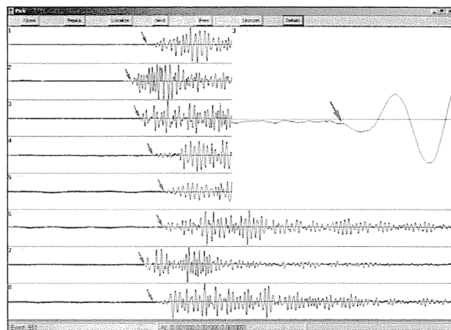
4. ábra: A nyolc szenzor által rögzített szignálok. A primer-hullámok belépésének meghatározása (nyilak) a WinPecker® programmal. Jobb fent segédablak a kurzor környezetének felnagyított képével.
