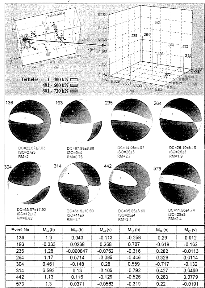
7. ábra: 1. csoport. Fent balra: a csoport elhelyezkedése, fent jobbra: a hangemissziós események heyezete a csoportban, középen: P-T-ábrák, lent: nyomatéki tenzor-komponensek
