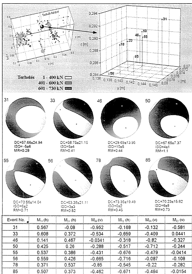
8. ábra: 2. csoport. Fent balra: a csoport elhelyezkedése, fent jobbra: a hangemissziós események helyzete a csoportban, középen: P-T-ábrák, lent: nyomatóki tenzor-komponensek
