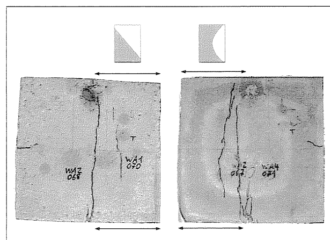
9. ábra: Ugyanazon próbatest szemben fekvő oldalai. A terhelt zóna (nyílak) alatti töréskép alapján nem dönthető el, hogy törési réteglap mentén való haránt irányú elcsúszás, vagy betonmorzsolódás következett be.
