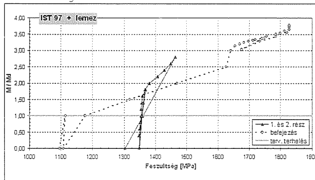
10. ábra: Az IST 97 pályalemezzel együttműködő gerenda próbaterhelési eredménye: relatív hajlító-nyomaték-pásmafeszültség diagram
