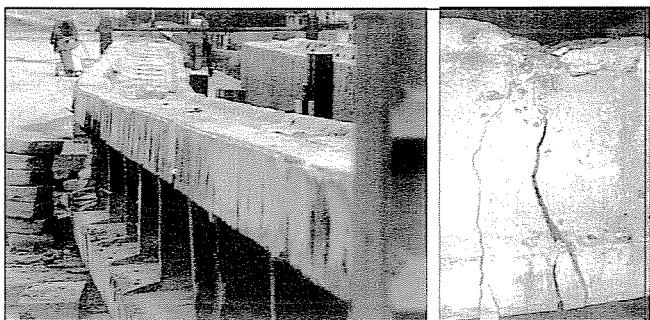
8. ábra: A VLOŠÁK tartók páros terhelési vizsgálat befejező fázisa (bal oldalon) és a tartó törésképe (jobb oldalon)
