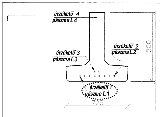
9. ábra: Az IST97: a pásmák és érzékelők számozása
