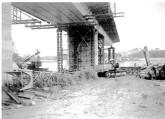
A lerombolt újvidéki Sloboda híd újjáépítése. (Ortortróp pályás szekrényes acél gerenda)
