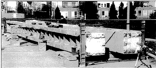
7. ábra: A VLOŠÁK tartók páros terhelési vizsgálatának előkészítési fázisa
