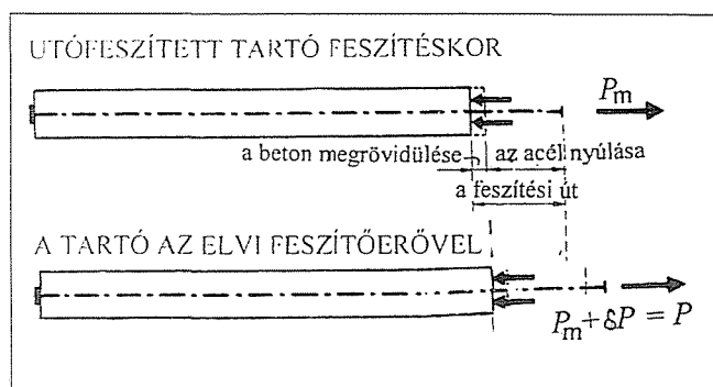
2. ábra: A definíció szerinti, elvi feszítőerő értelmezése utófeszített tartónál
