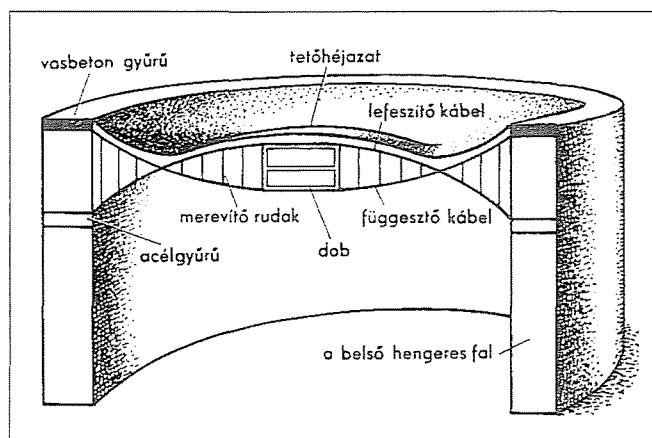
3. ábra: A kábelek elhelyezkedése (Ényedi, 1980)
