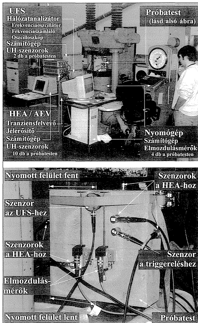
1. ábra: Kísérleti elrendezés
