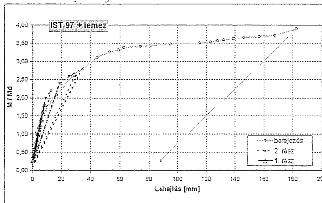
11. ábra: Az IST 97 pályalemezzel együttműködő gerenda próbaterhelése 1. és 2. szakaszának eredménye: relatív hajlító-nyomaték-lehajlás diagram
