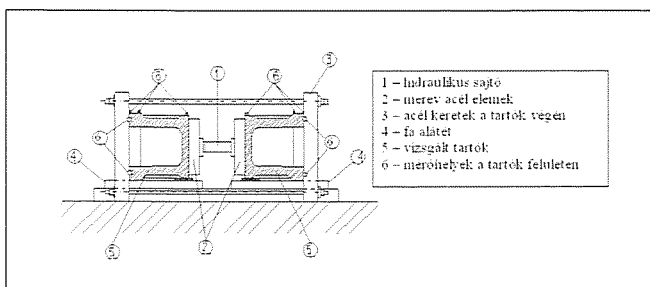
6. ábra: A VLOŠÁK tartók páros terhelése
