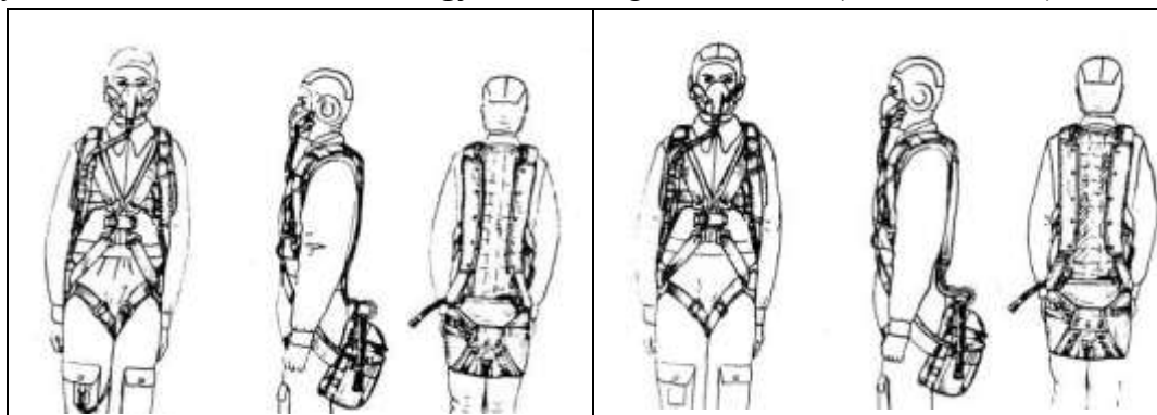
10. ábra Az Sz-3 típusjelzésű pilóta mentőejtőernyő általános nézete KP-23 vagy KP-27 ejtőernyős légzőkészülékkel, KAP-3 ejtőernyőnyitó félautomatával, MLASz-1 mentőcsónakkal. 44
