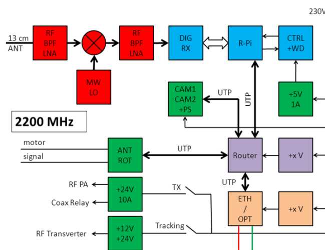
19. ábra A 2,2 / 2,4 GHz-es vevőág felépítése
