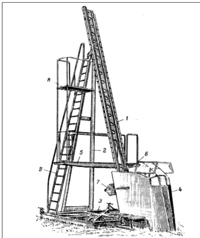
13. ábra A földi telepítésű NKTL-3 gyakorló katapult berendezés vázlata 24
