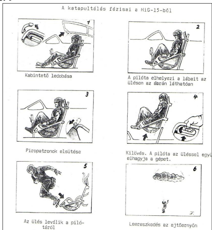
8. ábra A repülőgépvezetők részére készült vázlat a katapultálás végrehajtásának folyamatáról 13
