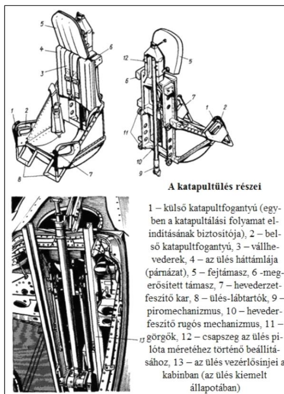
7. ábra A 1948-ban már sorozatgyártásra bocsátott katapultülés szerkezeti kialakítása 11
