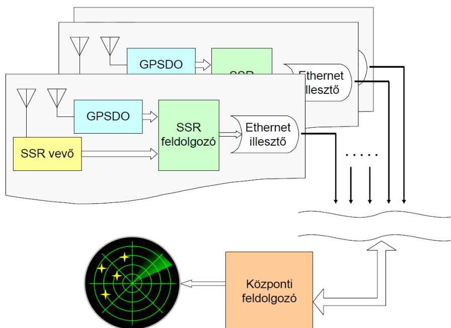
3. ábra Rendszer blokvázlat
