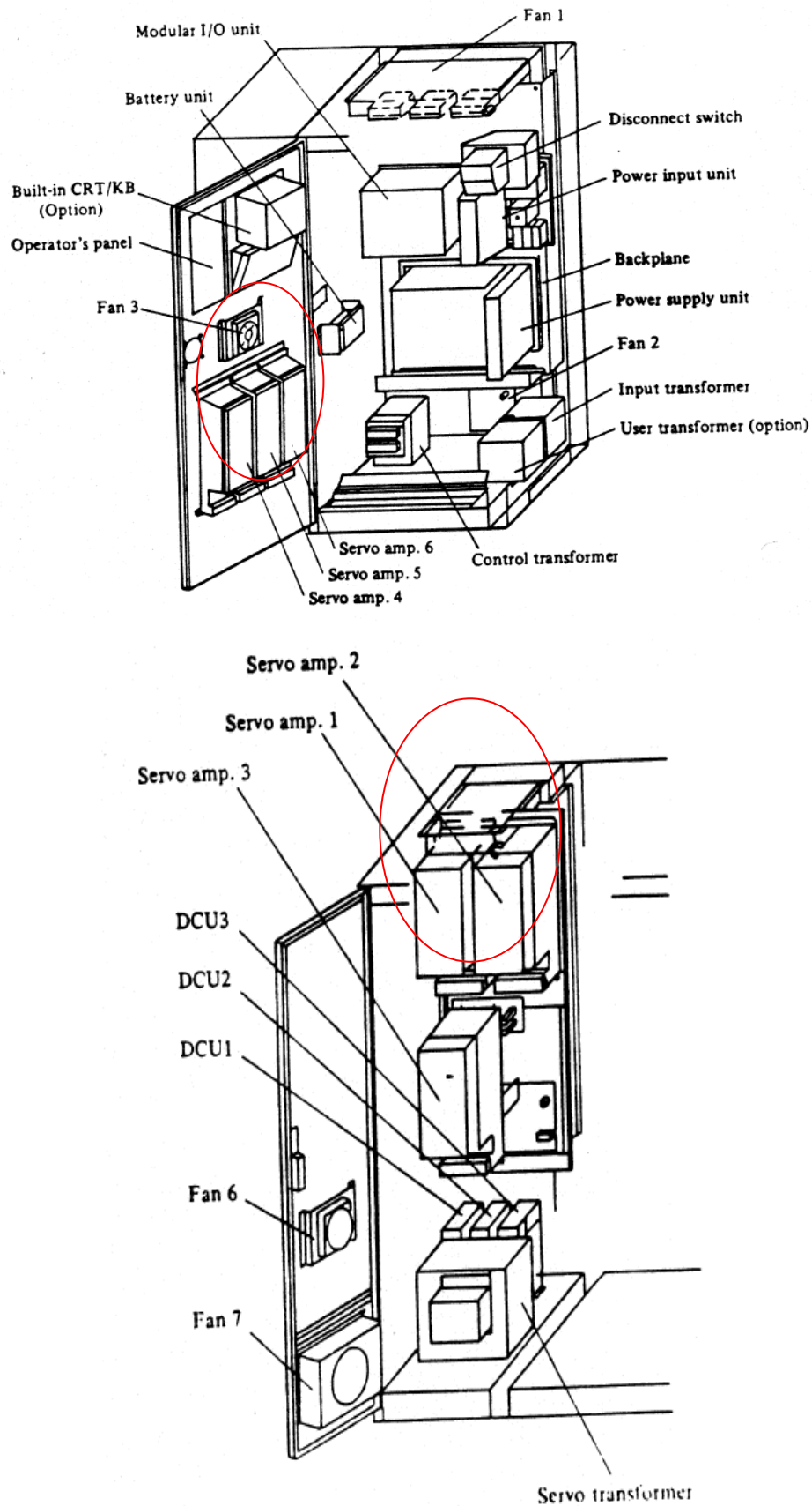
Fig. 1. FANUC S-420 Controller- Cabinet.
