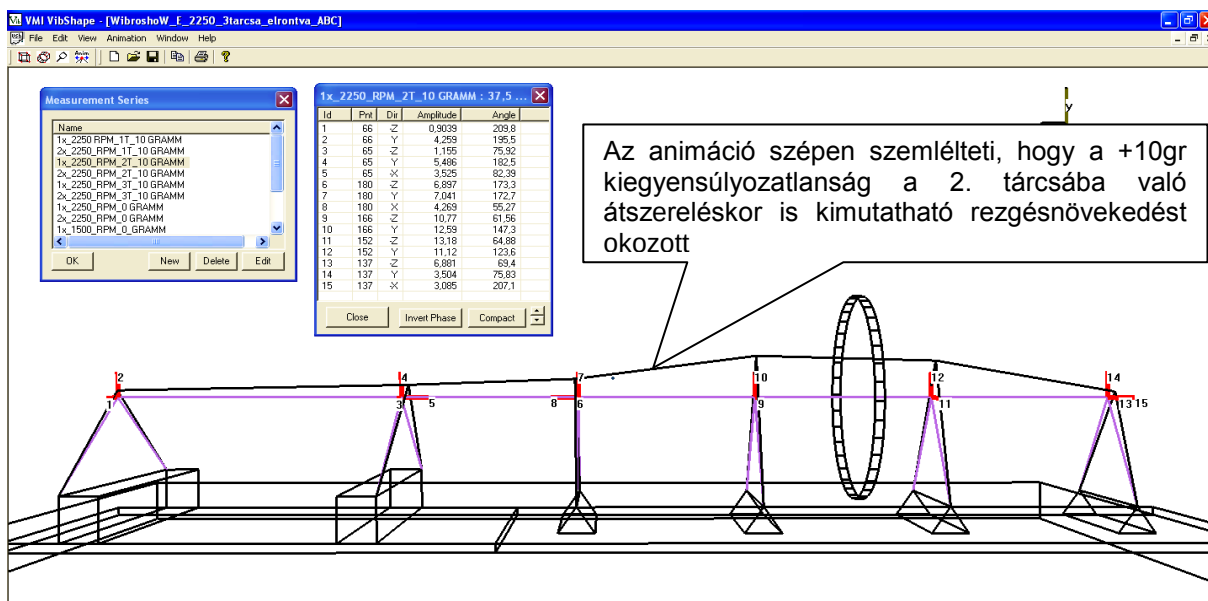
12. ábra. Az 5. animációs mérési sorozat eredménye 2250 1/min=37,5 Hz fordulatszámra jól látható, hogy az 2-es tárcsába szerelt +10 gr tömeg hatása, a rezgés „átvándorolt” 2 és 3 csapágyra
