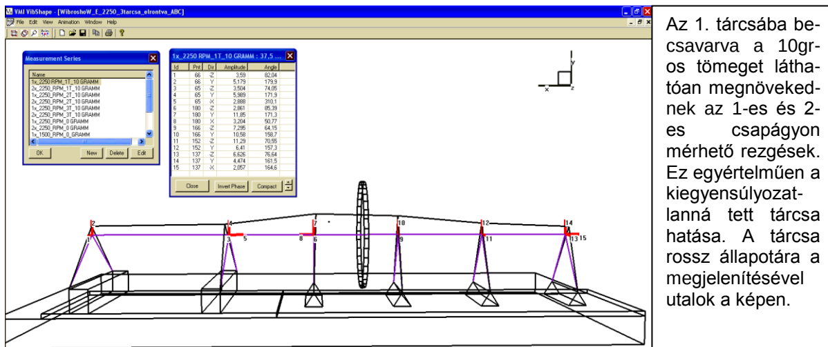
11. ábra. A 4. animációs mérési sorozat eredménye 2250 1/min=37,5 Hz fordulatszámra jól látható, hogy az 1-es tárcsába szerelt +10 gr tömeg hatására az 1 és 2 csapágyakon nőtték a rezgések
