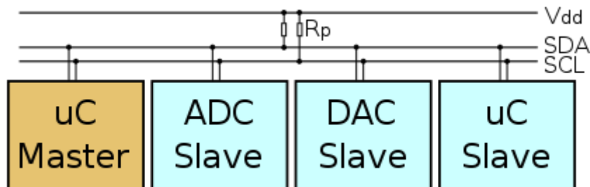
12. ábra. Az I 2 C kommunikáció vázlata [5]
