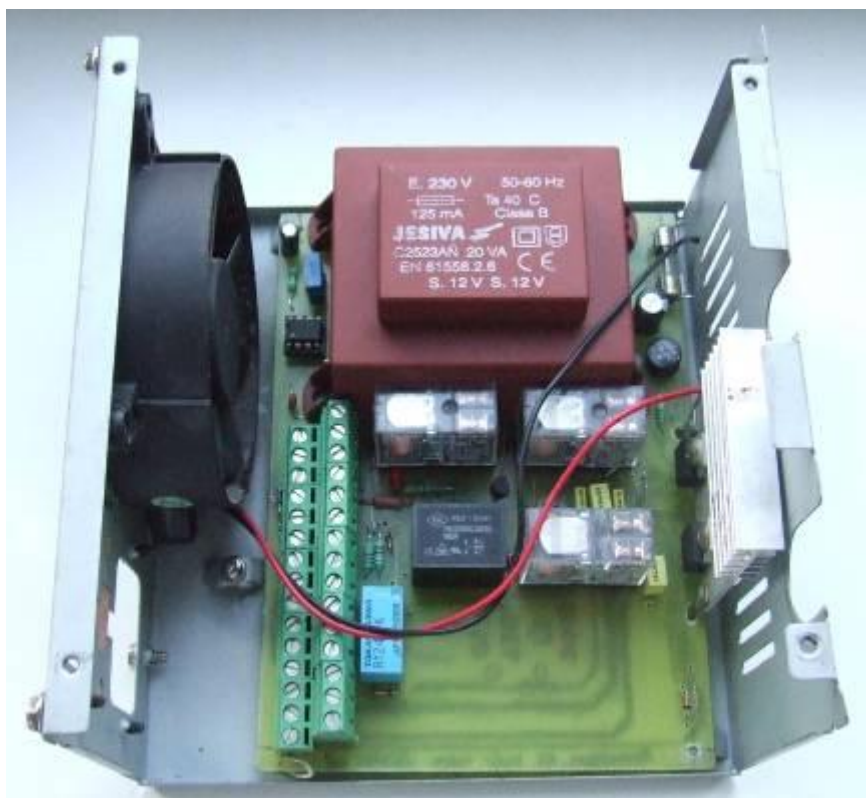
7. ábra: Az indító automatika
