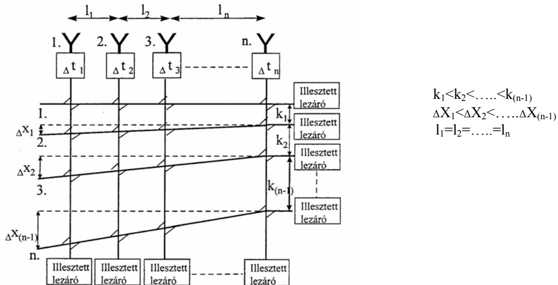
7. ábra Mátrix típusú nyalábeltérítés
