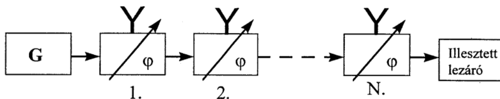
1. ábra Tápvonalszelekciós módszer
