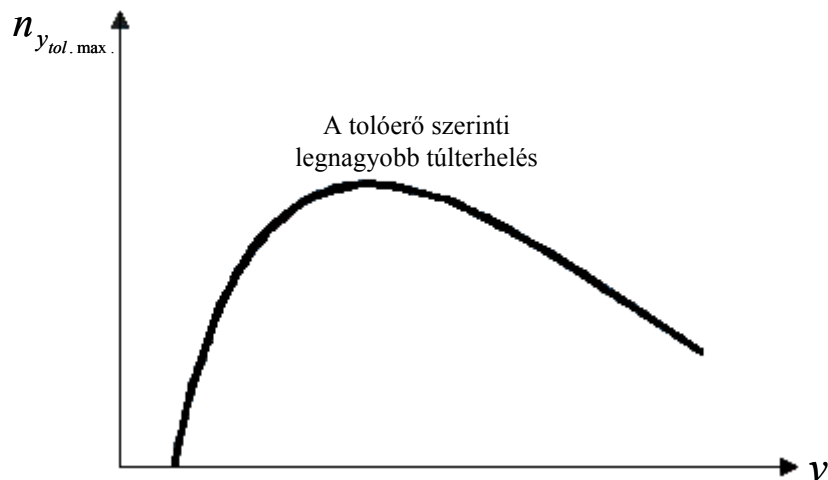
3. ábra. A repülőgép tolóerő szerinti maximális túlterhelése
