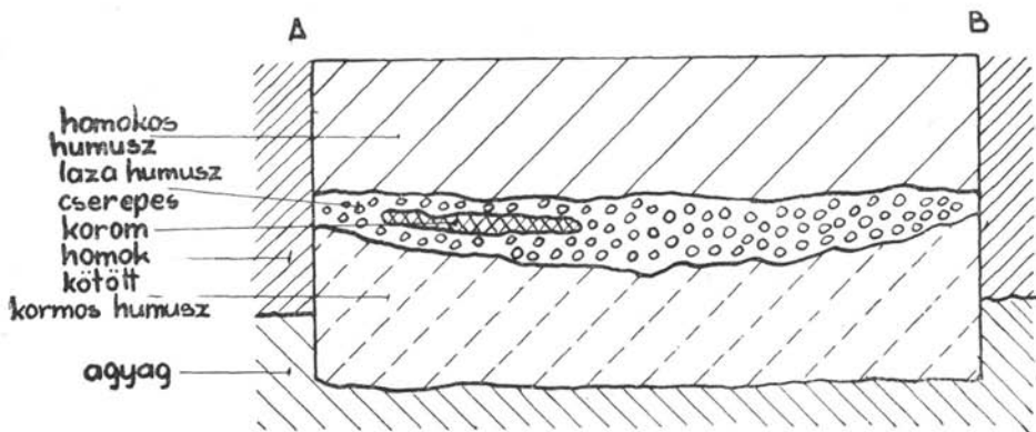
BOKROS-FEHÉRKERESZT Δ-B metszet
