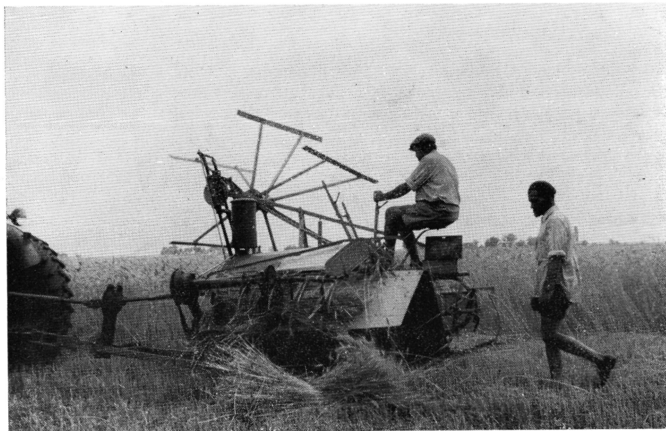
Aratógép munkaközben Žací stroj pri práci Erntemaschine während der Arbeit
