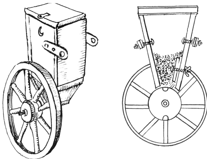
Ekére szerelhető kukoricapergető Na pluh pripevnená konštrukcia na siate kukurice Auf einen Pflug montierbarer Maissäer
