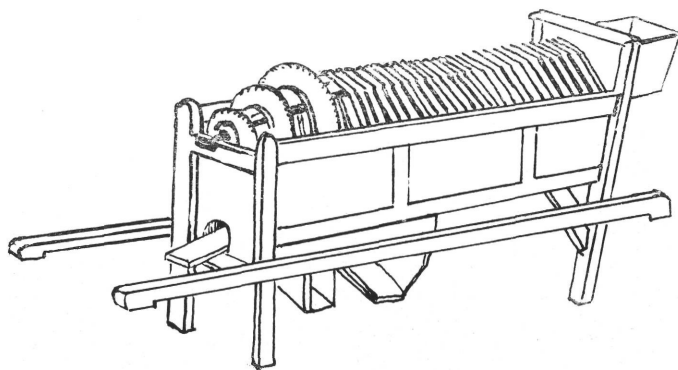
Hagymaosztályozó rosta Riečica na triedenie cibule Zwiebelssortier-Reiter
