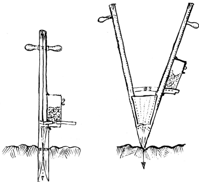
Kukoricaültető puska „Puška” na siatie kukurice Gerät zum Maissetzen ( puska )
