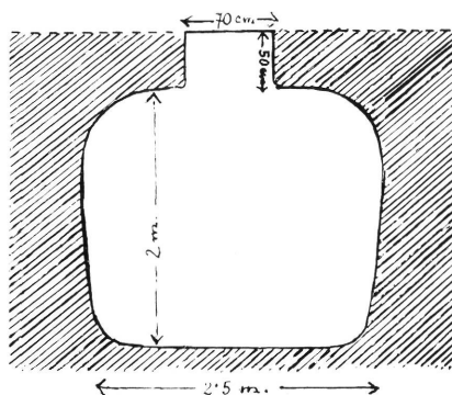
Gabonásverem Lehoczky Mátyás gazdálkodó elmondása szerint (rekonstrukció)
