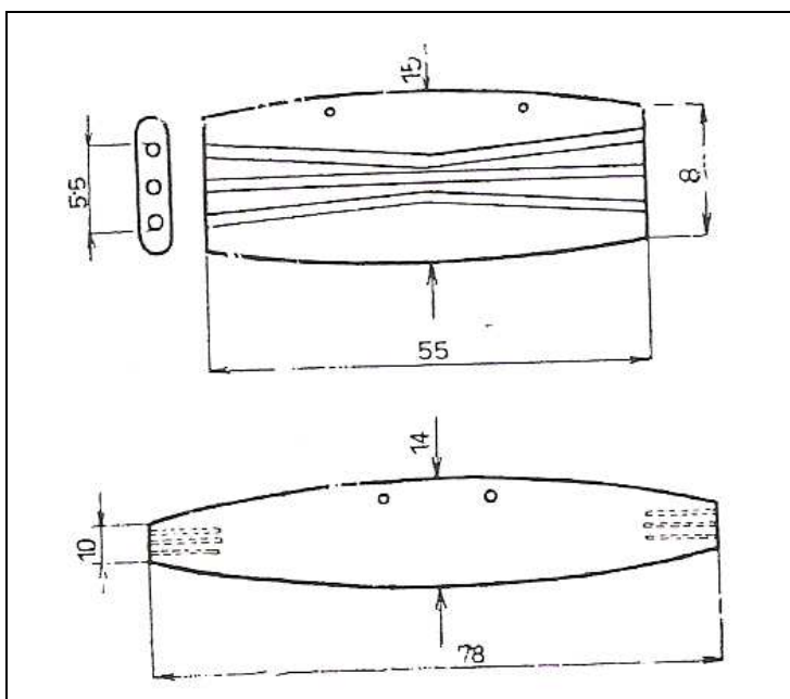
A lármafa kiviteli rajza. (FALLER Jenő, 1975. 155. nyomán.)
