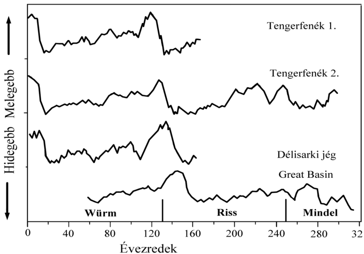
3. ábra. A Föld globális hőmérséklete és a jégkorszakok időrendje.
