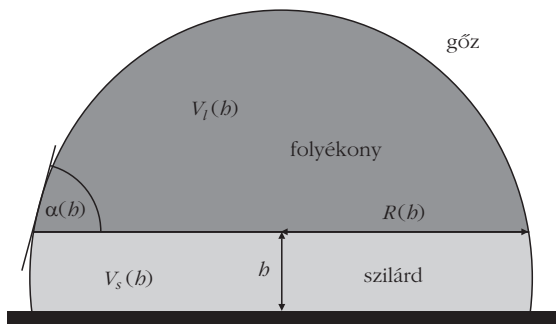
6. ábra. Megfagyó vízcsepp geometriája.
