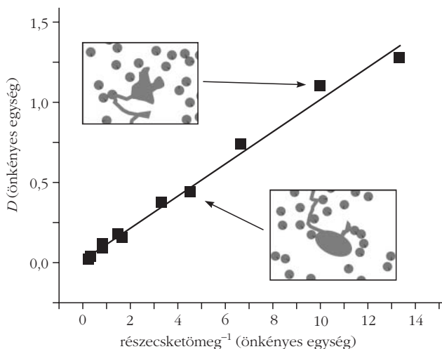
2. ábra. Különböző méretű és alakú szemcsék diffúziós együtthatójának alakulása a részecsketömeg reciprokanak függvényében.
