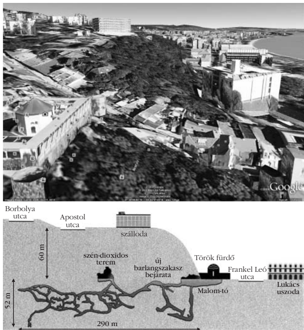
9. ábra. A József-hegy GoogleEarth által készített távlati képe, valamint a müontomográf helye és látószöge a 2. mérés során a Molnár János barlangban a József-hegy Ny–K irányú metszetén [13].
