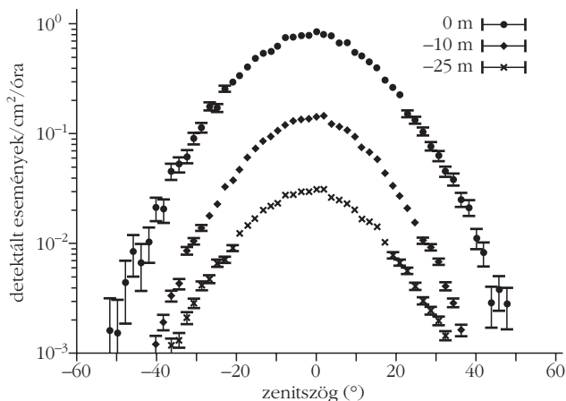
7. ábra. Müonhozam szögfüggése a földfelszínen, valamint 10 m és 25 m úgynevezett földkvivalens mélységeken.
