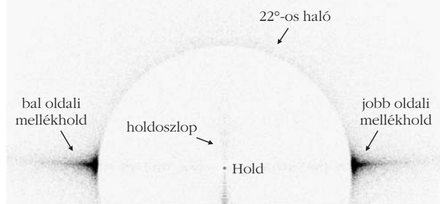
2. ábra. A modori és a szécsényi metszeten megjelenő holdhalók számítógépes szimulációja.
