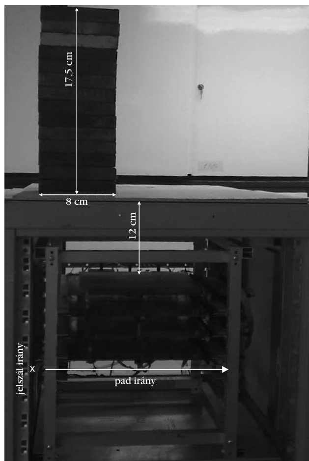
8. ábra. A müontomográf érzékenységét vizsgáló kísérleti összeállítás az ólomtoronnyal és az ólomtorony müonképevel.
