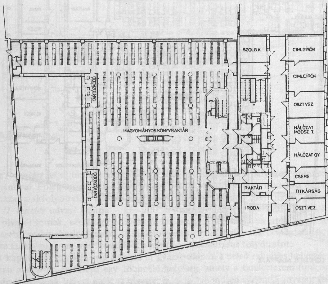
■ EMELETI ALAPRAJZ
