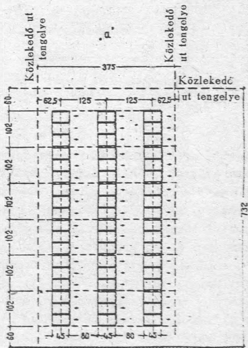
4a. ábra. A hagyományos, beépített kétoldalas állványokkal rendelkező könyvraktár átalakítása fiókos tárolásra (elrendezési vázlat).
