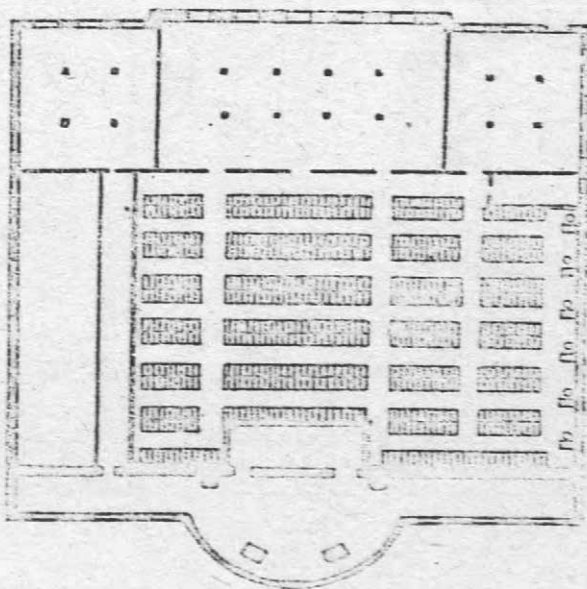
16. ábra. A Karélo-Finn ASzSzk petrozavodszki új közművelődési könyvtáráépületének tervezett raktára, kihúzható állványok tömör elrendezésével.
