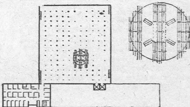
5. ábra. Tudományos könyvtár raktárának berendezése az egyik amerikai főiskola új épületében, tömören elhelyezett, ajtószerűen nyíló állványokkal
