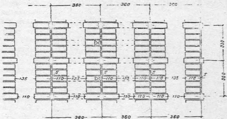
15. ábra. A Szovjetunió Tudományos Akadémiája új könyvtáráépületének tervében szereplő raktári elem vázlatos terve, kihúzható állványok tömör elrendezésével. (1939)
