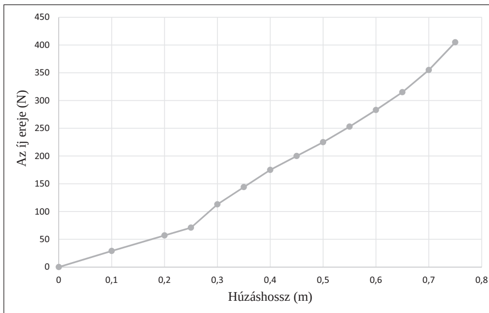
10. melléklet: IV. íj „A” erő-elmozdulás grafikonja hosszú ideg esetén
