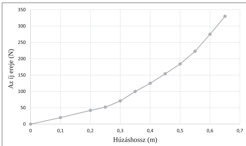
7. melléklet: Szkíta íj (I. íj) erő-elmozdulás grafikonja
