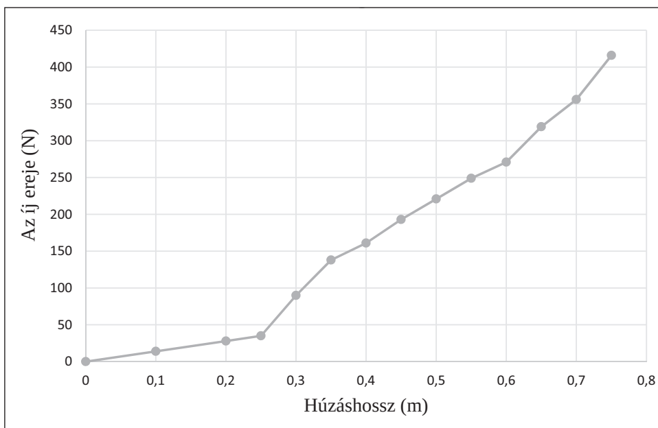
11. melléklet: IV. íj „B” erő-elmozdulás grafikonja rövidebb ideg esetén
