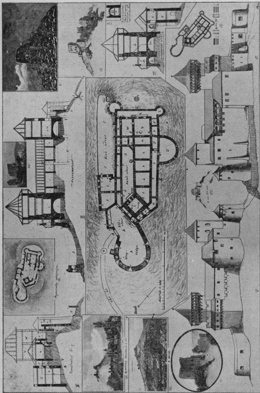
2. kép. — Torna vára. I. Alaprajz. II. Hosszmetézet. III. Keresztmetzet a palota mellett. IV. Keresztmetzet az öreg-tornyon át. V. Rekonstruált látkép délnyugat felől. VI. U. az északkelet felől. VII. Alaprajz Myskovszky szerint. VIII. Építési korok. IX. „R” pince keresztmetzete. X. A várom holdfényben kelet felől. XI. U. az nappal. XII. Az öregtorony délkelet felől. XIII. A tornai erődfített templom és a várhegy. XIV. A várhegy a várúttal (---). XV. Az öregtorony és a belső kapú helye. XVI. A várom a somodi—tornai országútról (délkelet felől).
